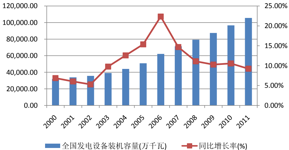
图 3 2000-2011 年全国发电设备装机容量
